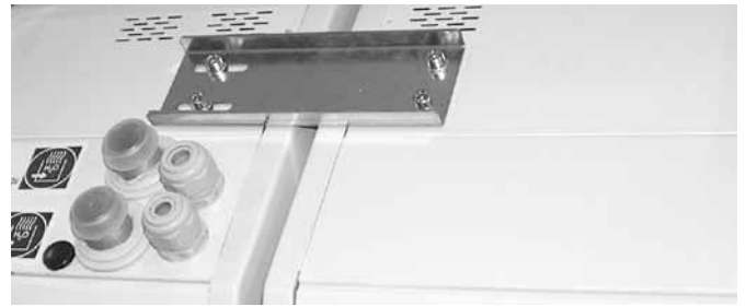
РИС. 23 – МЕХАНИЧЕСКОЕ СОЕДИНЕНИЕ ЗАВЕС C1
