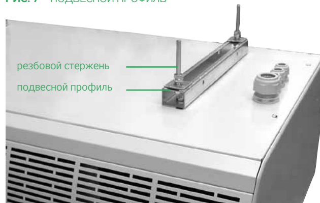
РИС. 7 – ПОДВЕСНОЙ ПРОФИЛЬ
