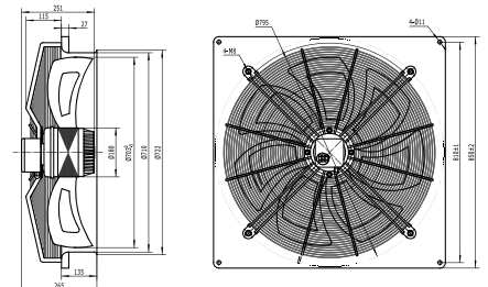
AXW 710-6D
