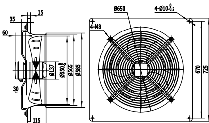
AXW 550-4D
