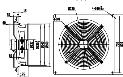
AXW 630-4D
