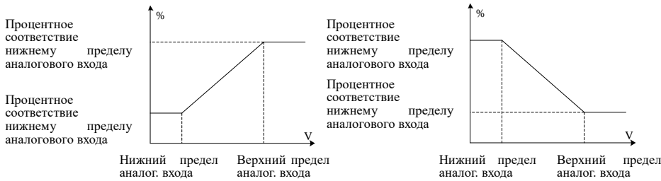
Рис. 6-18 Линейная кривая аналогового входа
