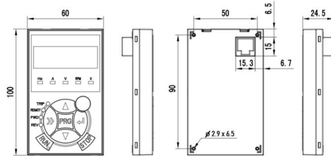
Рис.1-3 Схема пульта управления и монтажные размеры
