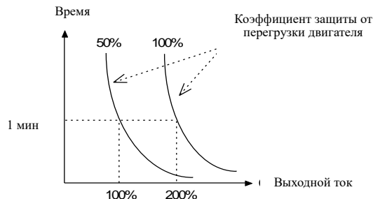
Рис. 6-27 Кривая защиты двигателя от перегрузки
